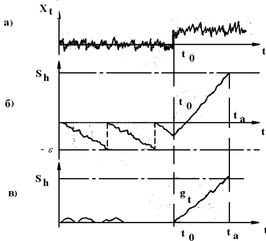
Рис. 1. Визначення моменту зміни статистичних властивостей часового ряду на основі використання АКС: а) розладка стаціонарного випадкового процесу в момент часу t_0 ; б) реалізація АКС (E. Page) з використанням ПКВЙ в) реалізація підходу А.Н.Ширяєва та G.Lorden до визначення АКС на основі обчислення статистики g_t з відбиваючим екраном.
