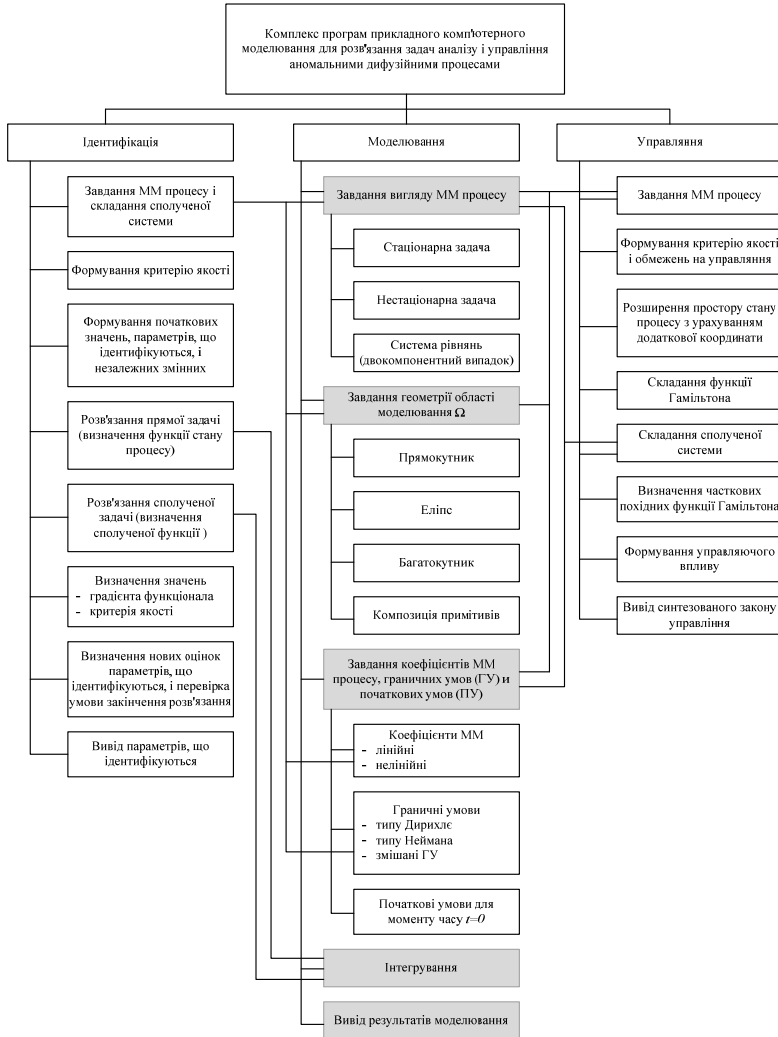
Рис. 1. Взаємозв'язок обчислювальних процедур при розв'язанні задач аналізу та управління
